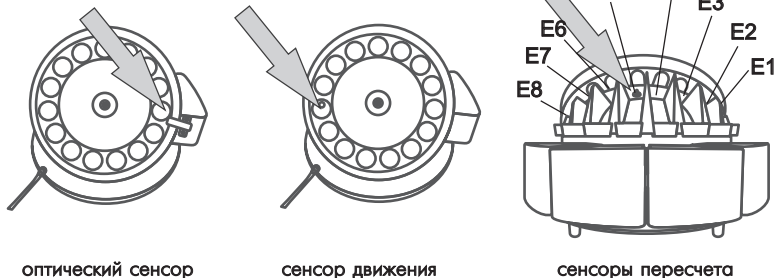
оптический сенсор
